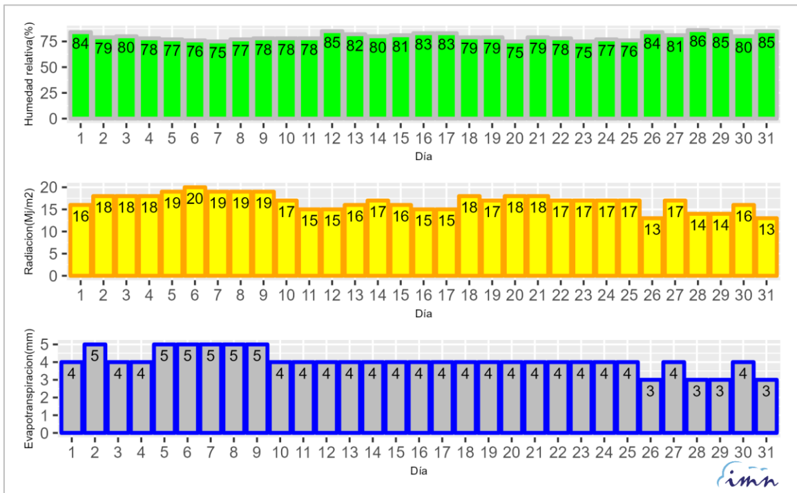
Figura 4.b. Promedio diario de humedad relativa (%), radiación solar (MJ/m²) y evapotranspiración referencia (mm) para octubre 2024 en la región arrocera Huetar Caribe
