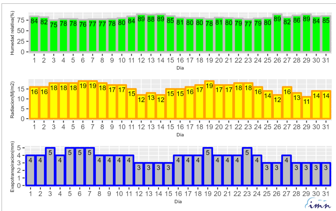
Figura 2.b. Promedio regional diario de humedad relativa (%), radiación solar (MJ/m²) y evapotranspiración referencia (mm) para octubre 2024 en la región arrocera Huetar Norte.
