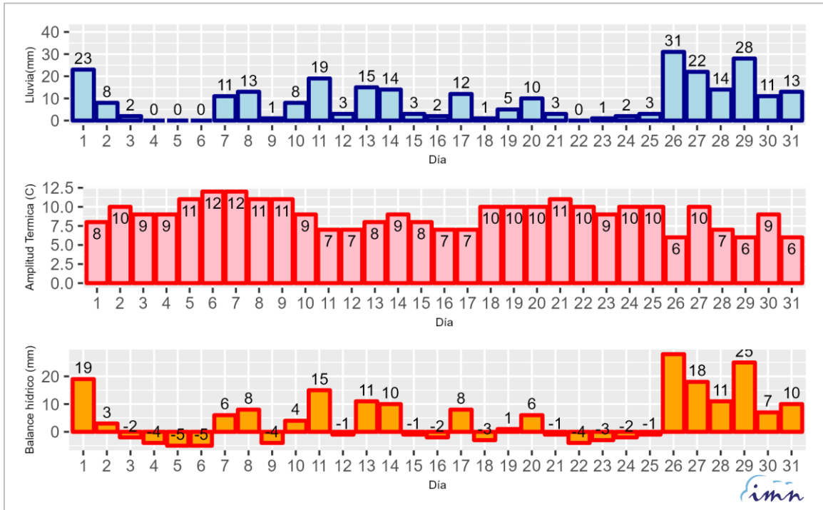
Figura 4.a. Promedio diario de precipitación (mm), amplitud térmica (°C), balance hídrico (mm) para octubre 2024 en la región arrocera Huetar Caribe
