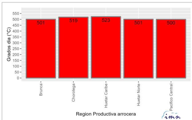
Figura 6. Grados día (°C) por región arrocera para octubre 2024 en la región arrocera.
