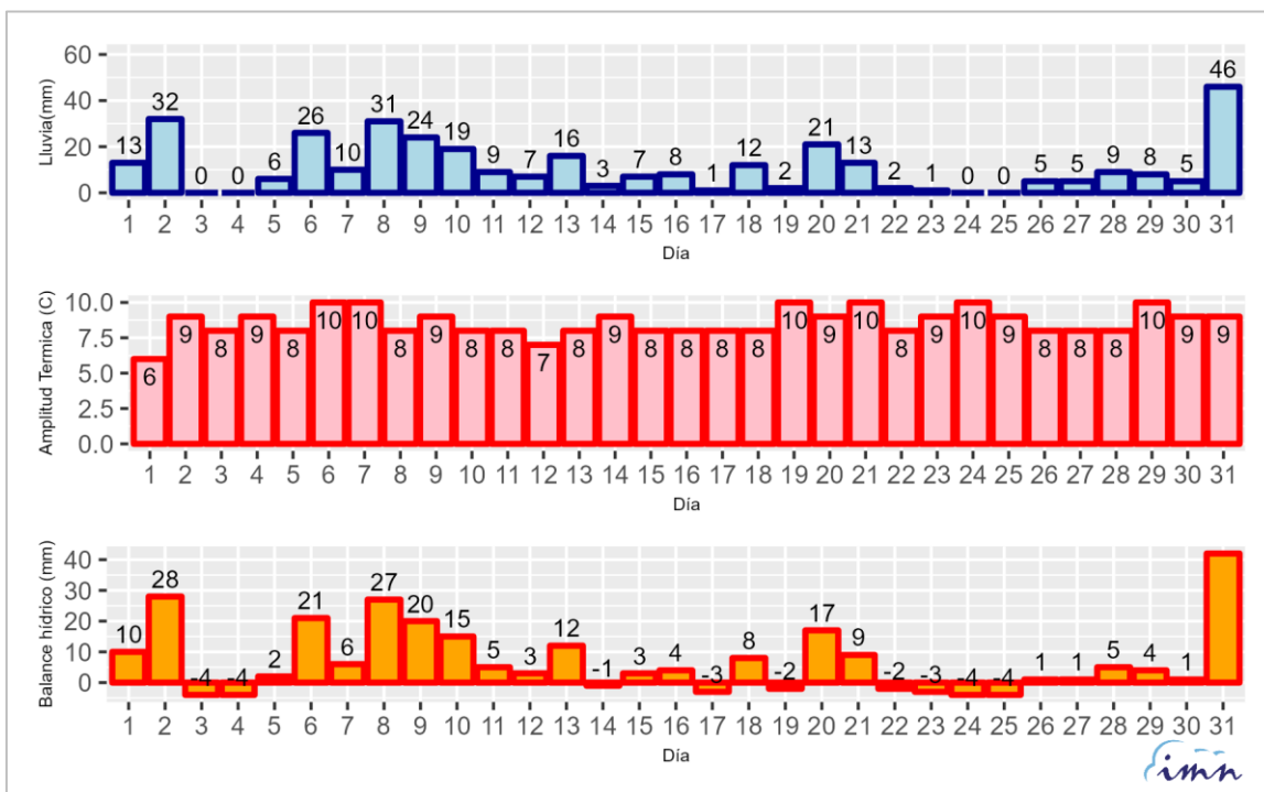
Figura 3.a. Promedio diario de precipitación (mm), amplitud térmica (°C), balance hídrico (mm) para octubre 2024 en la región arrocera Pacífico Central .
