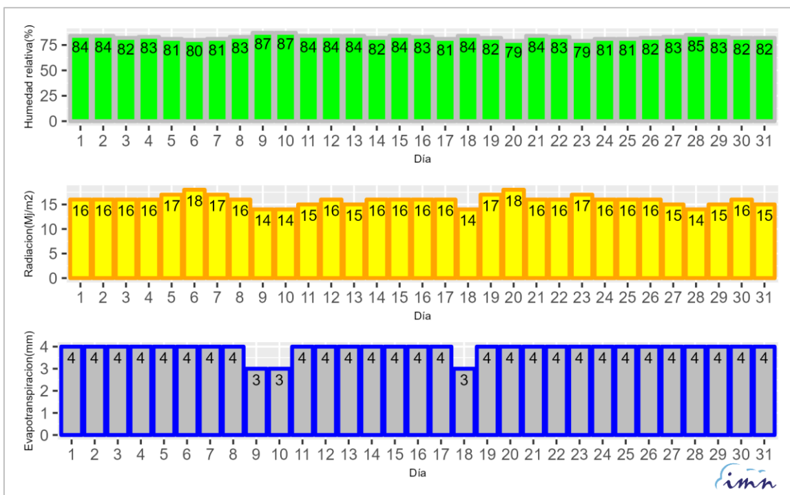
Figura 5.b. Promedio diario de humedad relativa (%), radiación solar (MJ/m²) y evapotranspiración referencia (mm)
