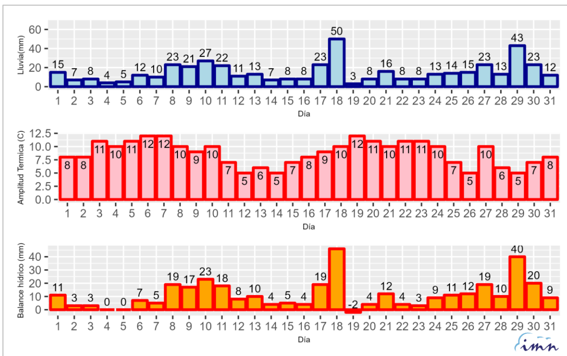
Figura 2.a. Promedio regional diario de precipitación (mm), amplitud térmica (°C), balance hídrico (mm) para octubre 2024 en la región arrocera Huetar Norte.
