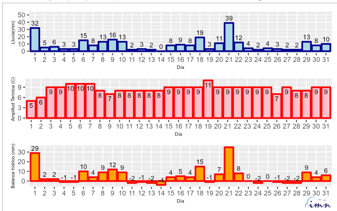
Figura 1.a. Promedio regional diario de precipitación (mm), amplitud térmica (°C), balance hídrico (mm) para octubre 2024 en la región arrocera Chorotega (Este y Oeste).
