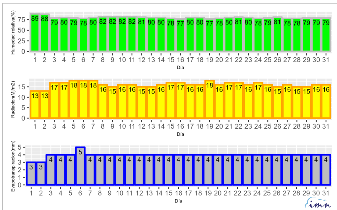
Figura 1.b. Promedio regional diario de humedad relativa (%), radiación solar (MJ/m 2 ) y evapotranspiración referencia (mm) para octubre 2024 en la región arrocera Chorotega (Este y Oeste).
