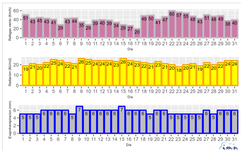
Figura 1.b. Promedio regional diario de viento máximo (Km/h), radiación solar (MJ/m²) y evapotranspiración referencia (mm) para marzo 2025 en la región cañera Guanacaste Este.
