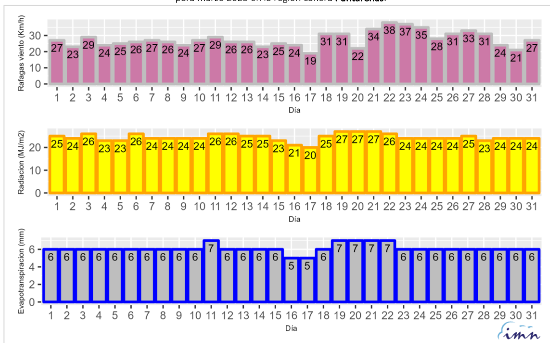
Figura 3.b. Promedio diario de viento máximo (Km/h), radiación solar (MJ/m²) y evapotranspiración referencia (mm) para marzo 2025 en la región cañera Puntarenas.
