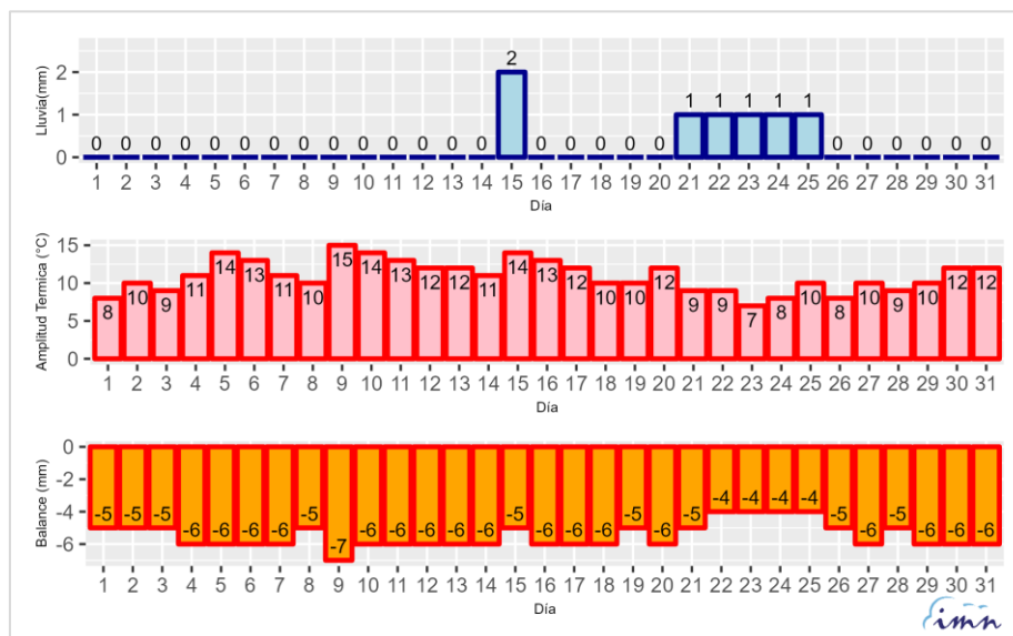
Figura 1.a. Promedio regional diario de precipitación (mm), amplitud térmica (°C), balance hídrico (mm) para marzo 2025 en la región cañera Guanacaste Este.
