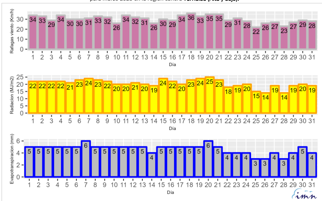
Figura 6. Promedio diario de viento máximo (Km/h), radiación solar (MJ/m²) y evapotranspiración referencia (mm) para marzo 2025 en la región cañera Turrialba (Alta y Baja).
