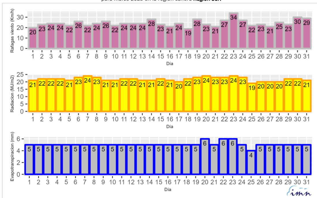
Figura 7.b. Promedio diario de viento máximo (Km/h), radiación solar (MJ/m²) y evapotranspiración referencia (mm) para marzo 2025 en la región cañera Región Sur .
