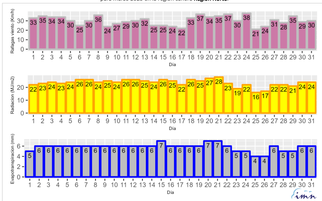
Figura 4.b. Promedio diario de viento máximo (Km/h), radiación solar (MJ/m²) y evapotranspiración referencia (mm) para marzo 2025 en la región cañera Región Norte .
