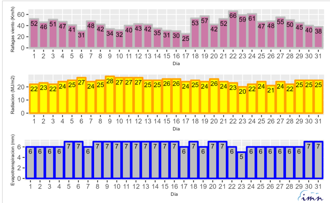
Figura 2.b. Promedio regional diario de viento máximo (Km/h), radiación solar (MJ/m²) y evapotranspiración referencia (mm) para marzo 2025 en la región cañera Guanacaste Oeste .
