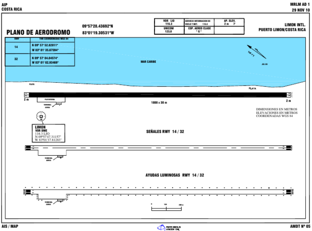
FIGURA 5 Plano de aeródromo de MRLM. Adaptado de [2].
